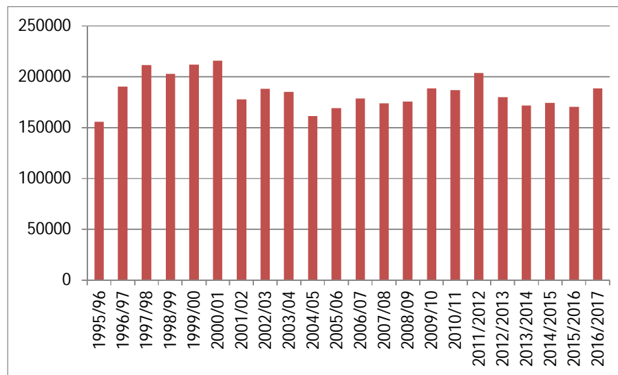
Figuur 1: Aantal veediefstalsake wat aangemeld is
